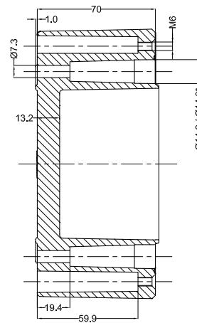
SECTION D-D
