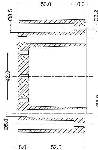
SECTION D-D
