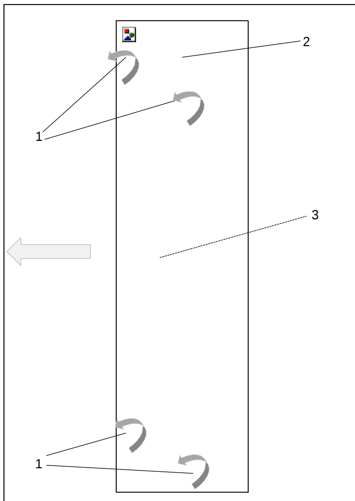
Abbildung 17 – Gerätehaube demontieren
