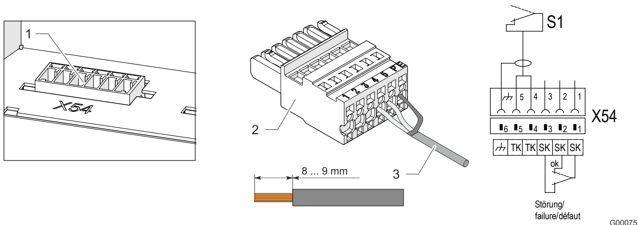
Fig. 17: Conexión del interruptor de contacto de puerta
