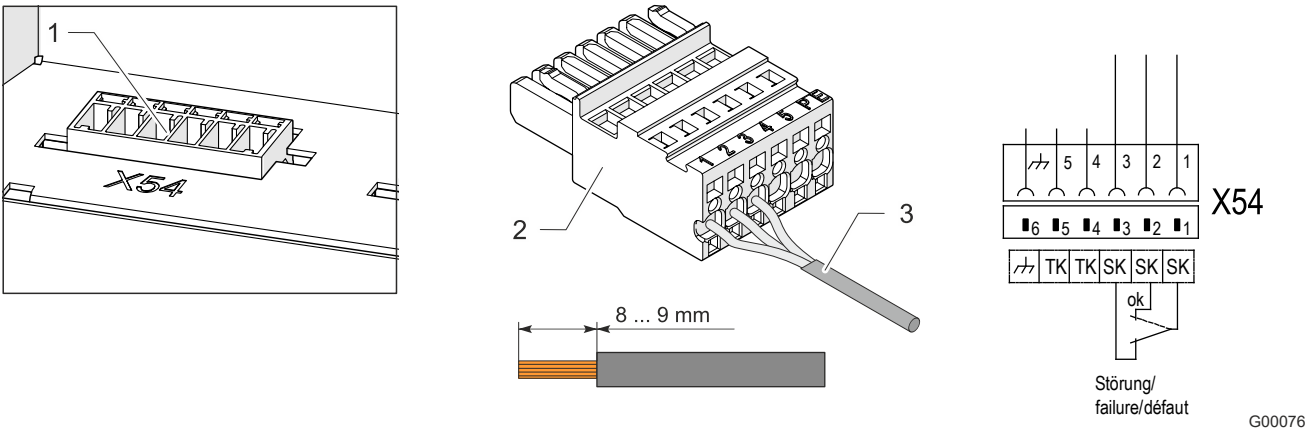
Abb. 18: Sammelstörmeldung anschließen (Beispiel)
