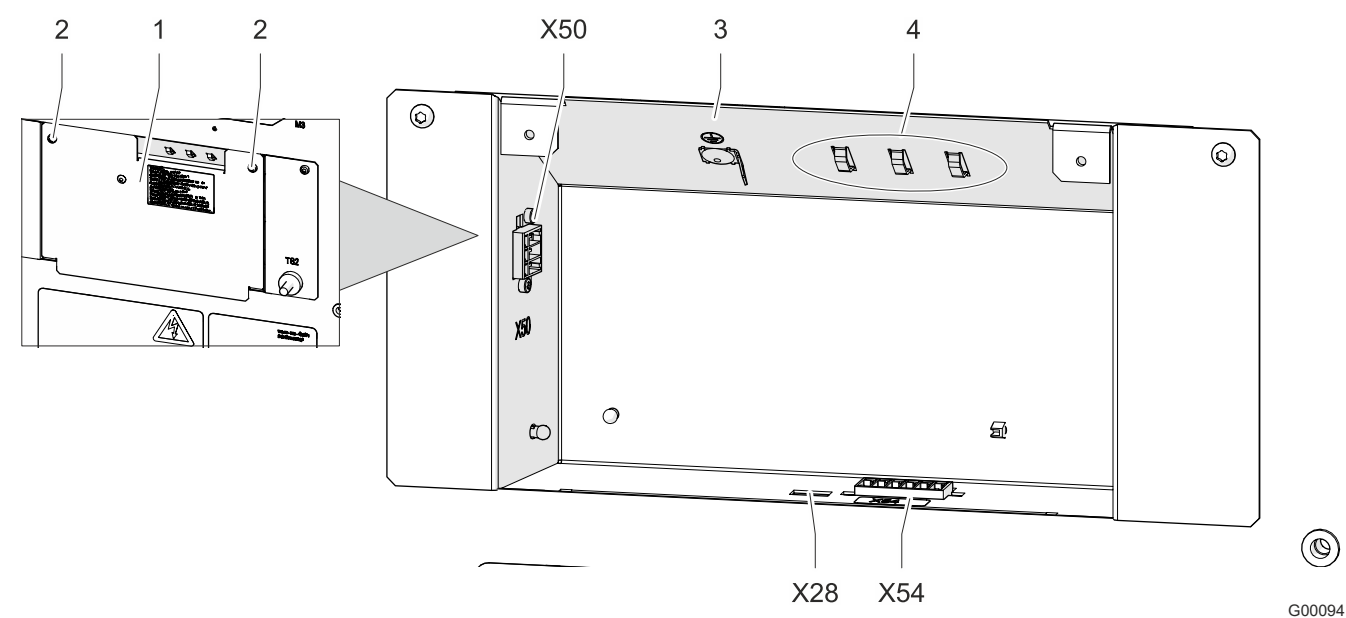
Fig. 15: Área de conexión
