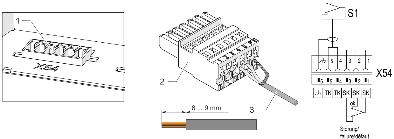
Abb. 17: Türkontaktschalter anschließen
