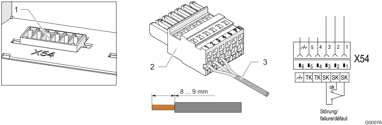
Fig. 18: Collegare il messaggio di guasto cumulativo (esempio)
