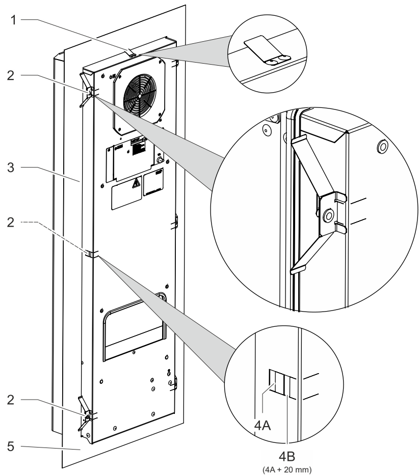
Fig. 13: montage du climatiseur
