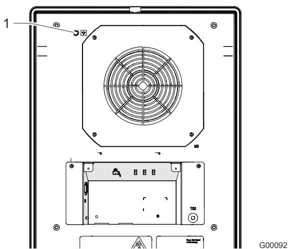
Fig. 20: Conexión equipotencial
