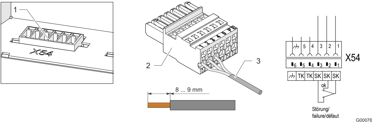
Рис. 18: Подключение сообщения о групповой ошибке (пример)
