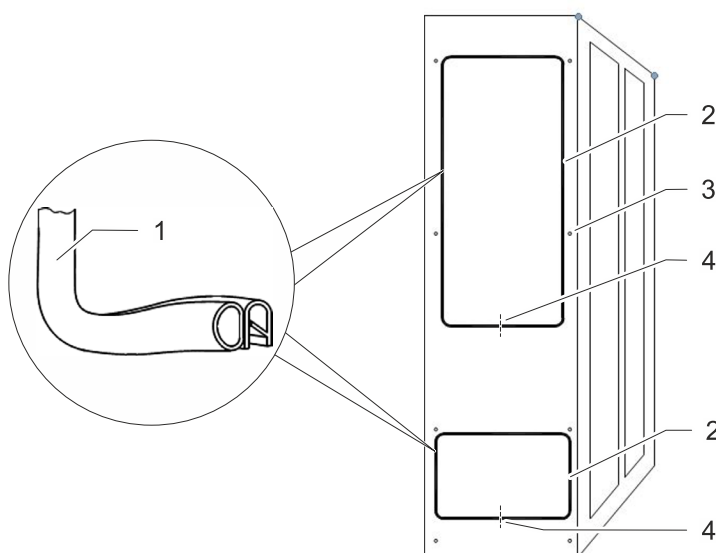
Рис. 11: Установить профильное уплотнение
