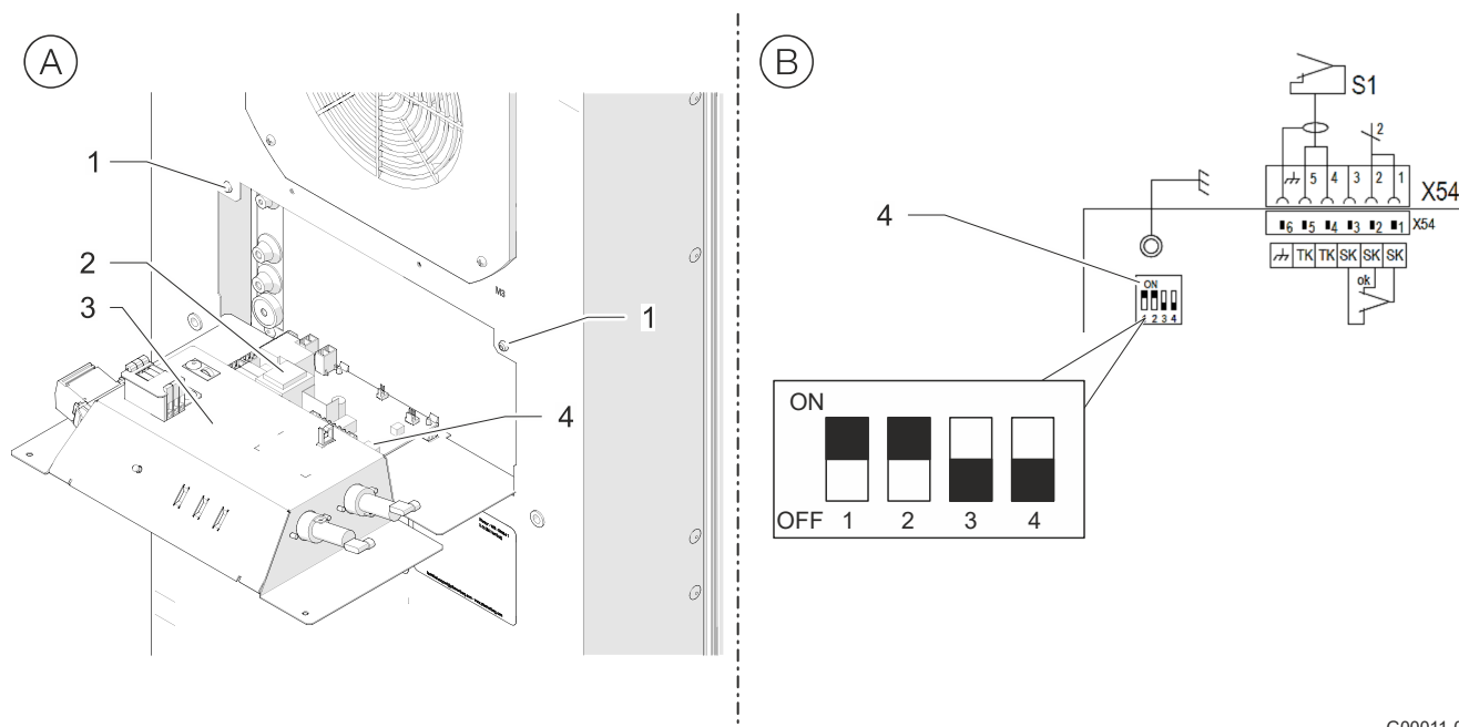
Abb. 16: DIP-Schalter einstellen
