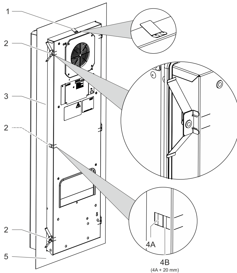
Abb. 13: Kühlgerät montieren
