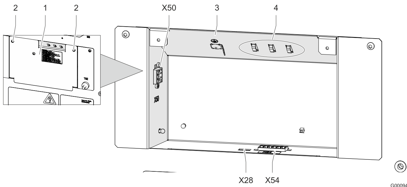
Рис. 15: Коммутационный отсек
