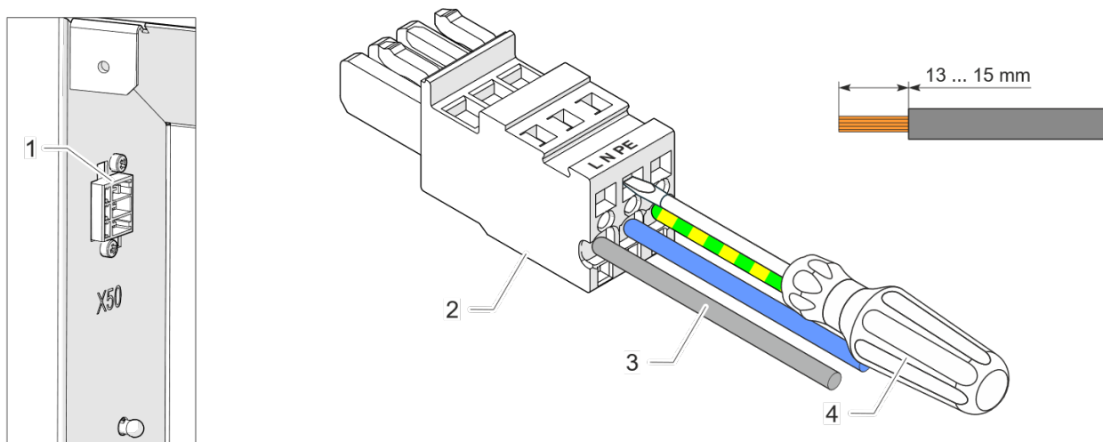
Fig. 19: Connettore di collegamento alla rete del condizionatore
