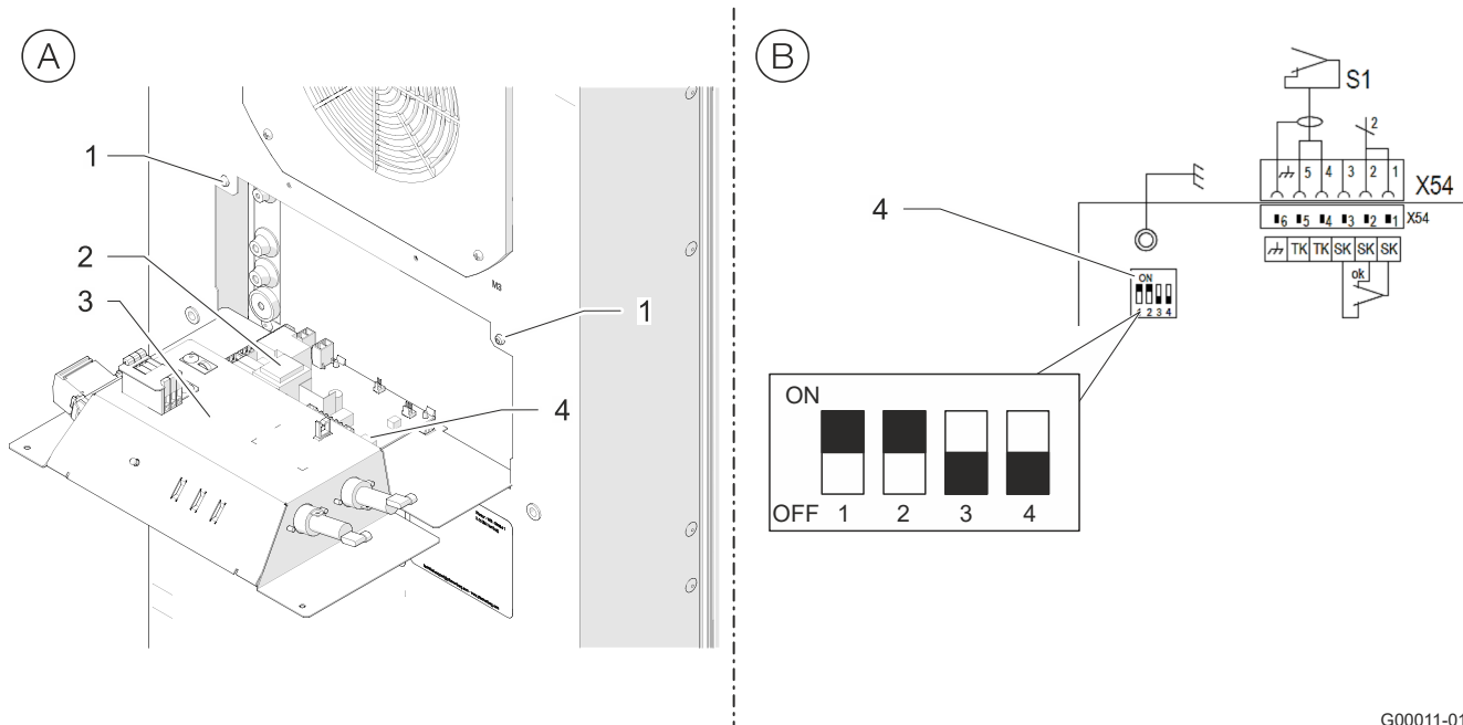
Рис. 16.: Настройка DIP-переключателя
