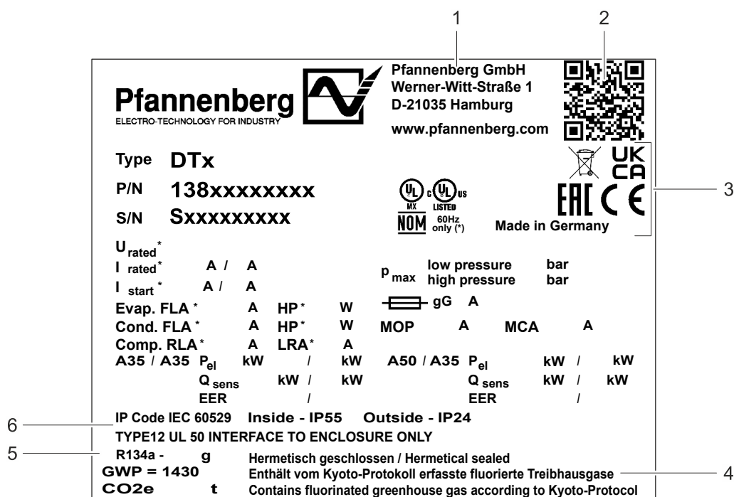
Abb. 8: Typenschild (Beispiel)
