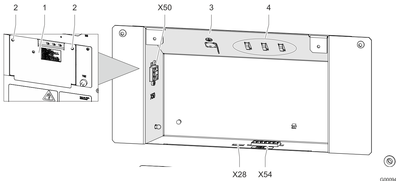
Abb. 15: Anschlussraum
