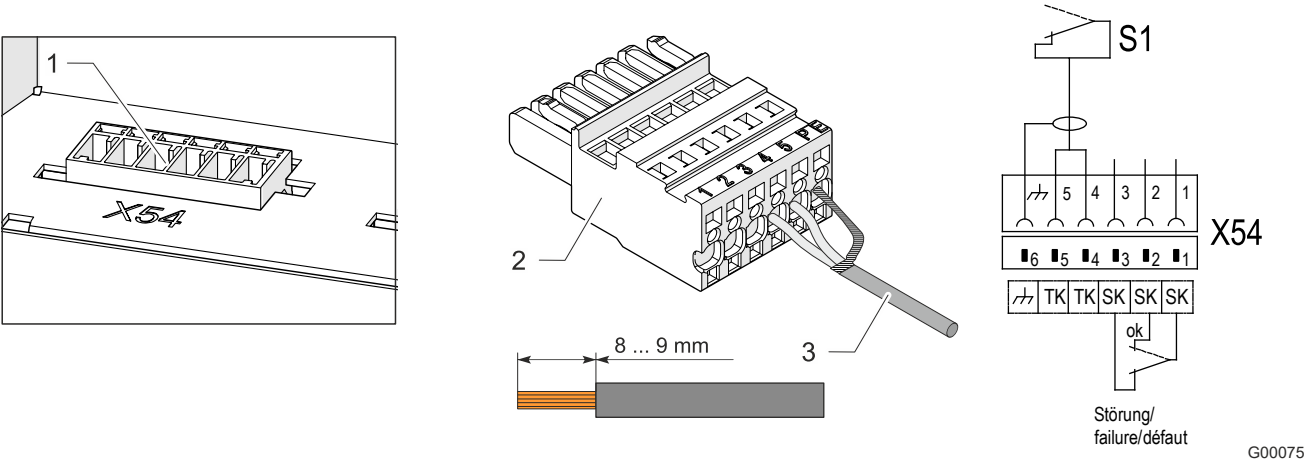
Рис. 17: Подключение дверного контактного выключателя
