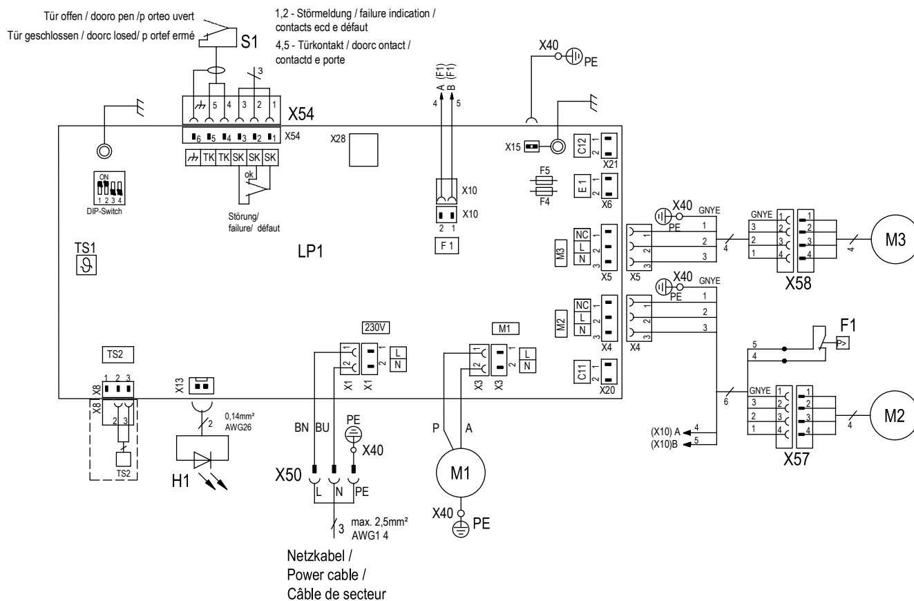
Fig. 14: Schema elettrico
