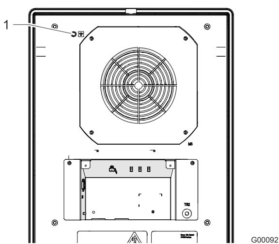
Fig. 20: Equipotential bonding
