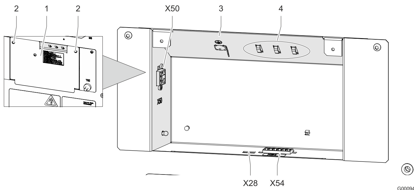
Fig. 15 : compartiment de raccordement
