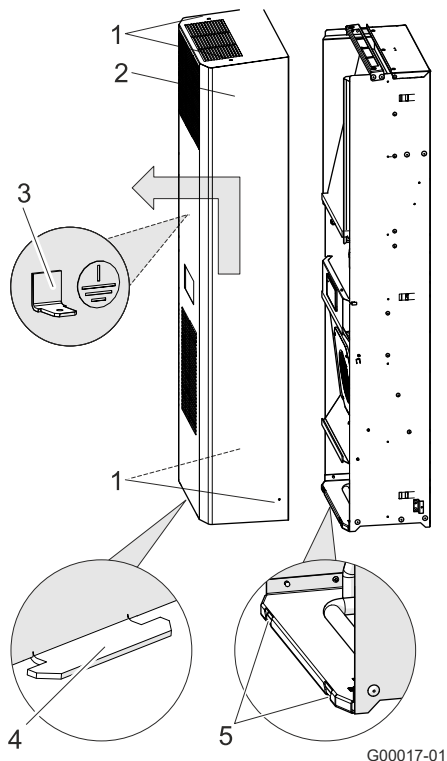
Fig. 23: Smontaggio del coperchio dell'apparecchio
