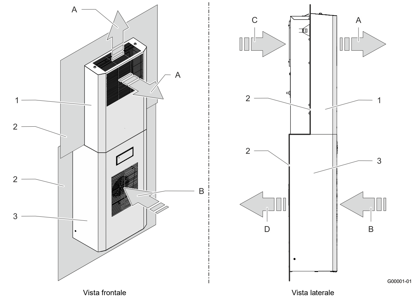
Fig. 3: Circuito di ventilazione quadro elettrico DTI/DTS
