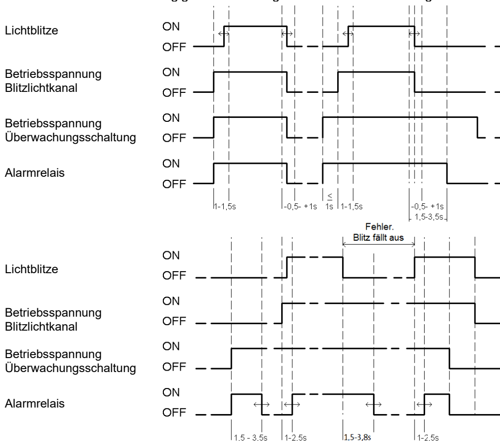
Abb. 9 Funktions-Zeitdiagramm
