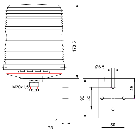
Abb. 4 Gesamtansichten
