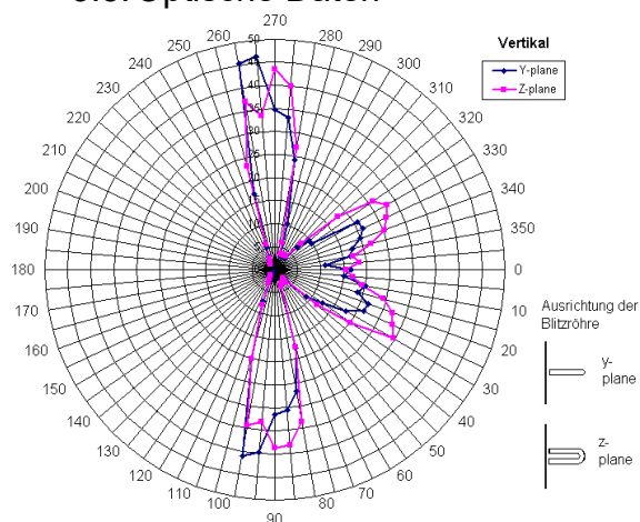
Abb. 5 Richtdiagramme
